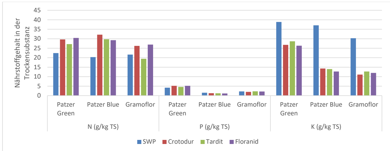
Abb. 2: Nährstoffgehalt in der Trockensubstanz der Zonal-Pelargonien zum Versuchsende (LfULG Dresden-Pillnitz 2022)
