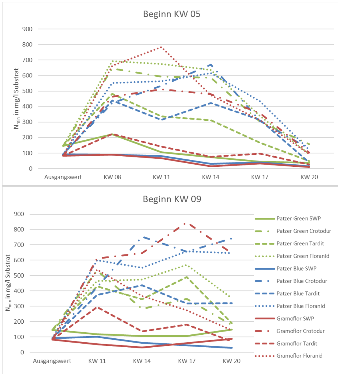
Abb. 1: Verlauf der N_{min} -Gehalte im Substrat in den beiden Kultursätzen ab KW 05 und ab KW 09 bei Zonal-Pelargonien (LfULG Dresden-Pillnitz 2022)
